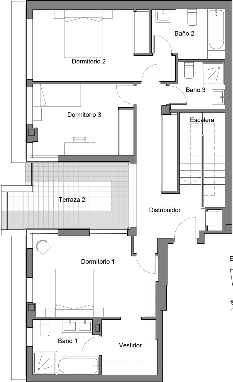
PLANTA 3ª
