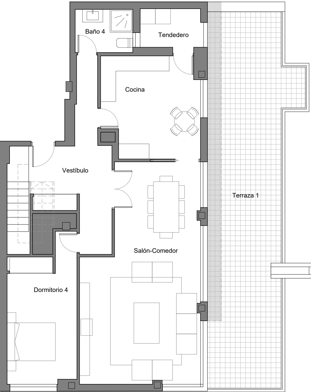
PLANTA 2ª
